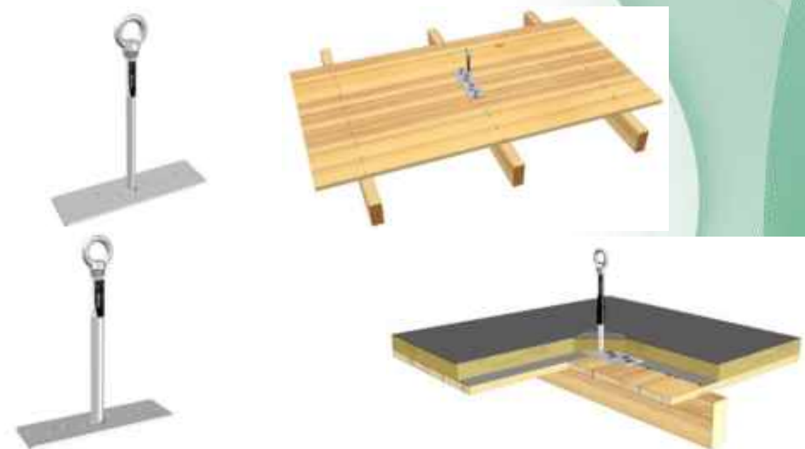
Bilder 30 - 33: LUX-top® ASP EV 7
