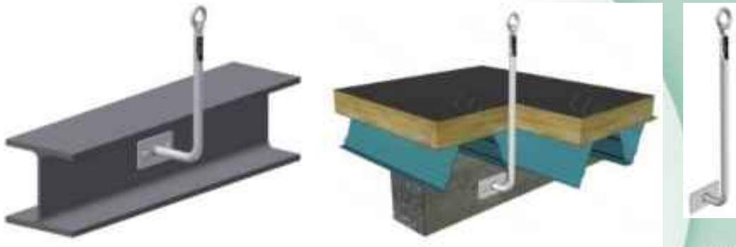
Bilder 10 – 12: Anschlagereinrichtung, Typ: LUX-top® ASP EV 2s 90°
