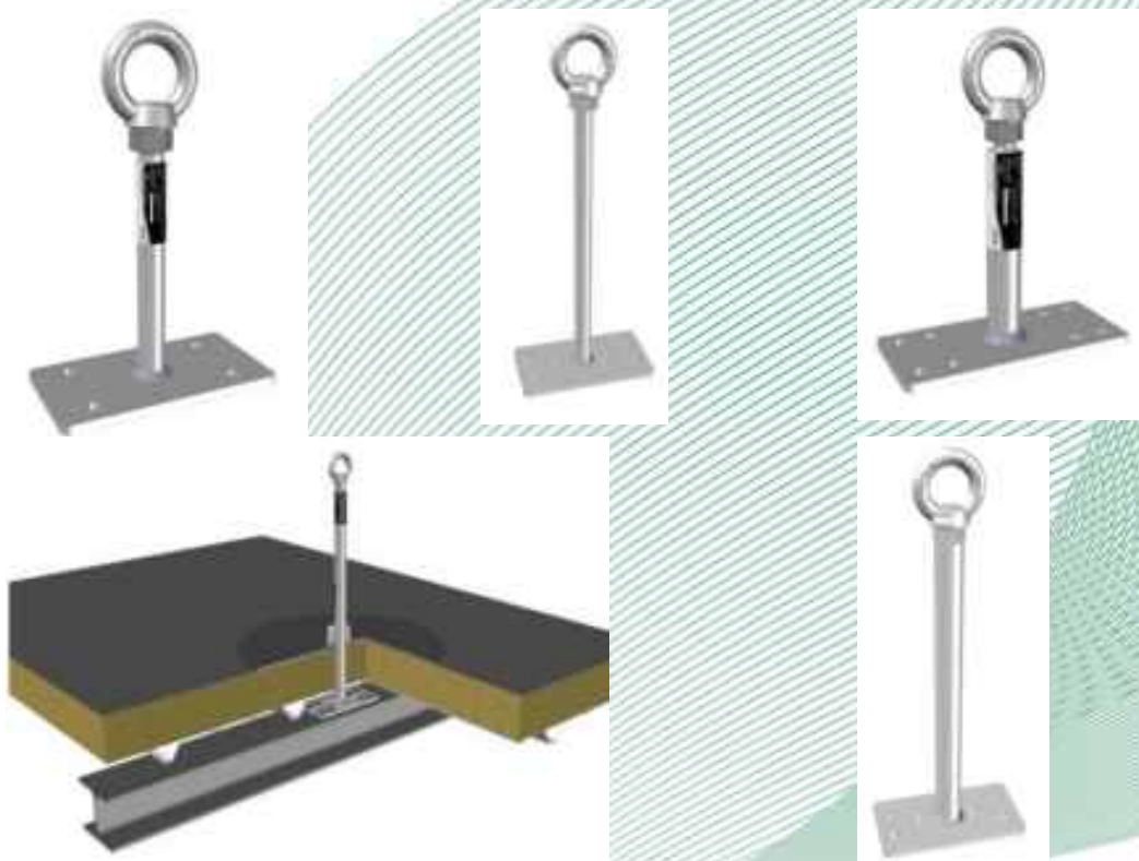
Bilder 15 – 19: Anschlagereinrichtung, Typ: LUX-top® ASP EV 4s
