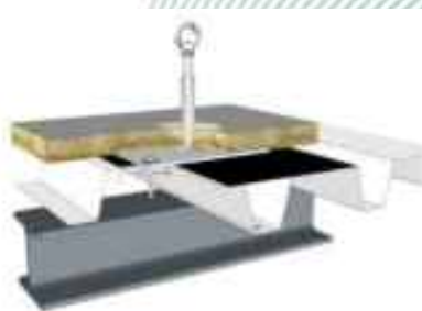
Bilder 46 – 48: LUX-top® ASP EV 9 II
