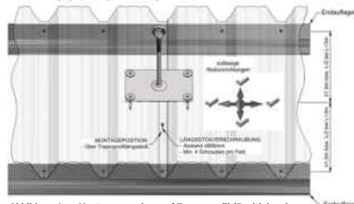
Abbildung 1a – Montagevorgaben auf Trapezprofil (Positivlage) bei Absturzrichtung quer zur Trapezprofilspannrichtung
