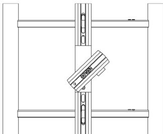
Abb.13 Bsp. drehbare Entnahmeklappe
