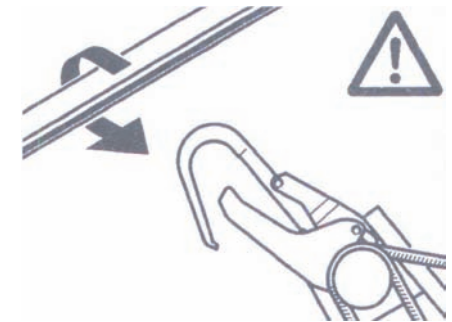
A Rohrhaken mit der Fernbedienstange am Anschlagpunkt oberhalb des Verunglückten einhängen.
