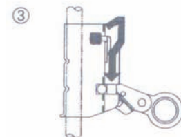
Seilklemme verriegelt automatisch. Verriegelung prüfen!
