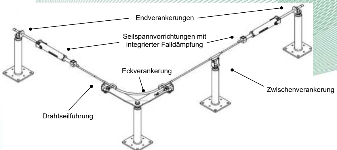
Bild 1: Anwendungsbeispiel der Anschlageinrichtung, Typ: ALLinONE
